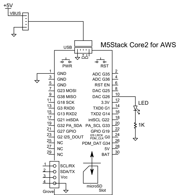
M5Stack Core2 for AWS Lチカ 電気回路図
